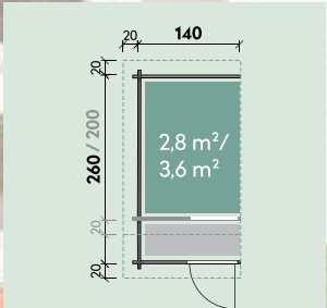
Anbauschuppen 1420/1426
