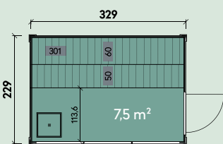
Stina 3323/1-Raum
