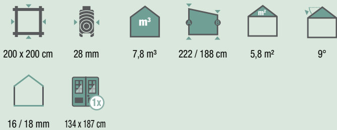
Luca 2020 Art.-Nr. 228277
