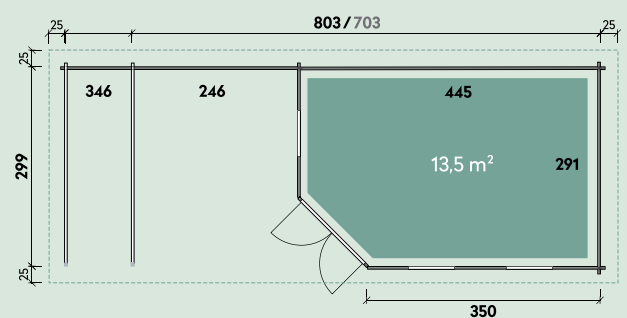
Melinda 7030 / Melinda 8030
