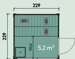
Stina 2323/1-Raum
