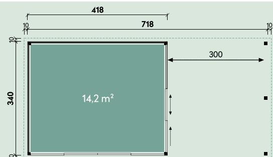
Isabell 7234
