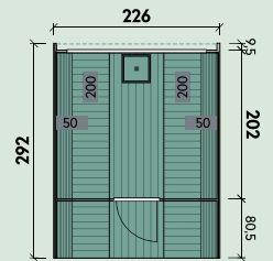
FREIJA 2329
