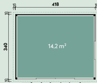
Isa 4234
