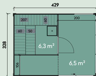
Stina 4333/2-Raum
